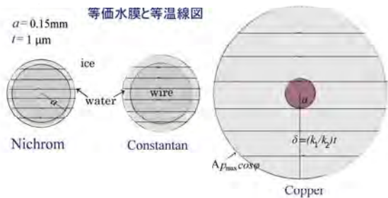
図 4.23 ワイヤー熱伝導率に等価な等価水膜図
