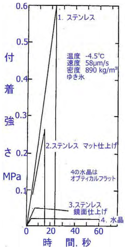
図 3.44 単位面積当たりのせん断付着力と時間との関係(Jellinek)
