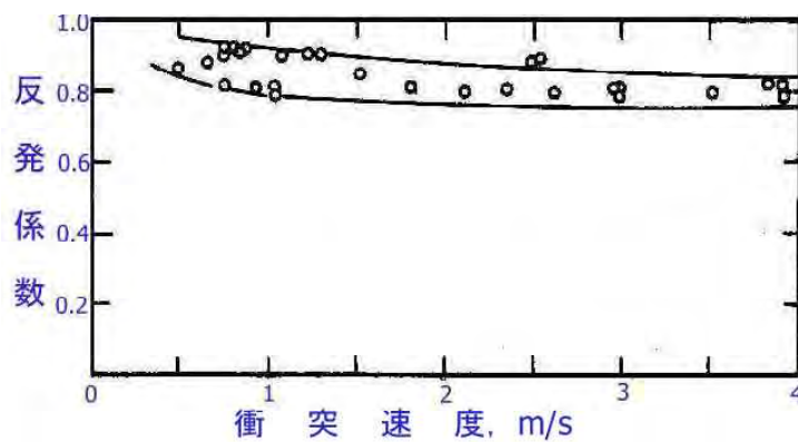
図 3.58 水平板と氷球の衝突 (低温科学,1978)
