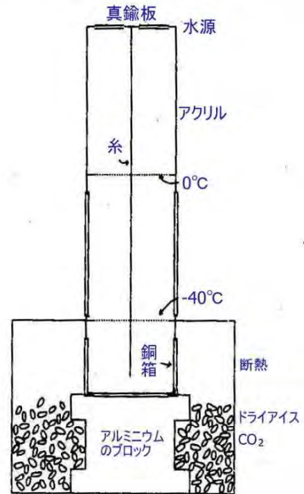
図 5.32 拡散式人工雪作成法
