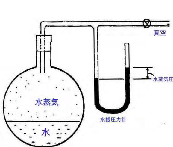
図 4.29 水蒸気圧の測定
