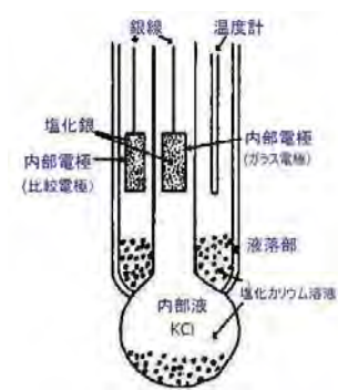
図 8.16 pH メーター
