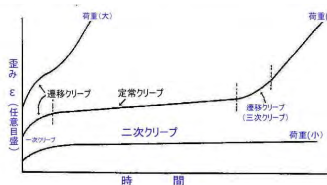
図 3.17 氷のクリープ曲線
