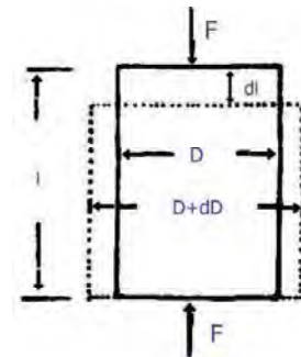
図 2.20 縦方向の縮みと横方向の広がり
