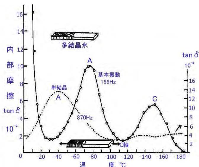
図 3.32 氷の内部摩擦の温度依存性（黒岩・山地，1959） 実線（多結晶氷）は左側目盛，破線（単結晶氷）は右側目盛
