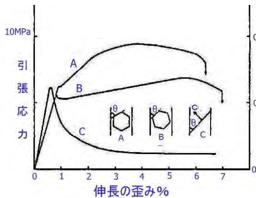
図 3.20 単結晶氷の定速度圧縮
