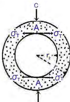
図 3.22 引っ張り破壊
