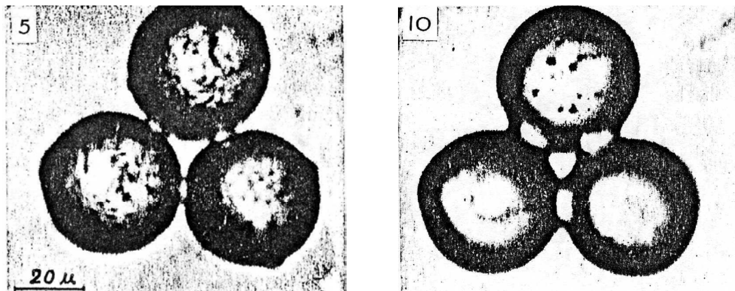
図 4.14 ケロシン(灯油)中での氷球の焼結 左は開始 35 分後、右は 1369 分後(黒岩, 1960)
