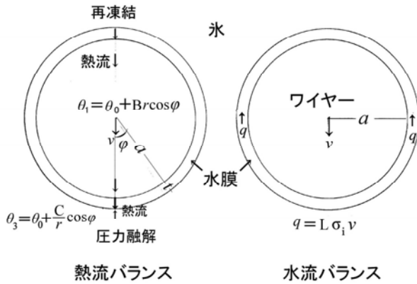
図 4.22 熱流バランスと水流バランス
