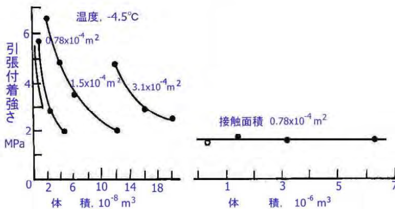
図 3.37 付着体の氷の体積と付着強さ(Jellinek, 1953)
