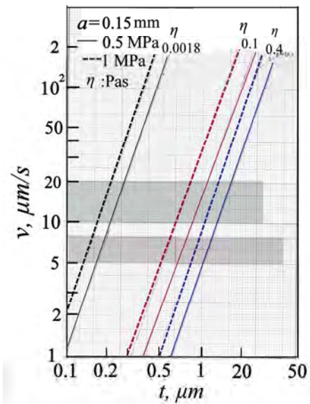
図 C.1 水膜の粘性係数と貫入速度
