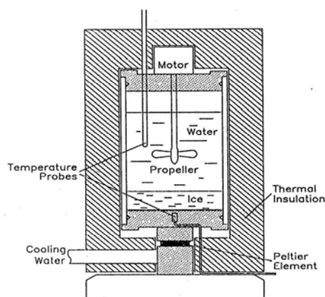
図 8.2 水・氷間の分別係数の測定 (M.Lehmann & U.Siegenthalen J.Glaciol.Vol.37,1991)
