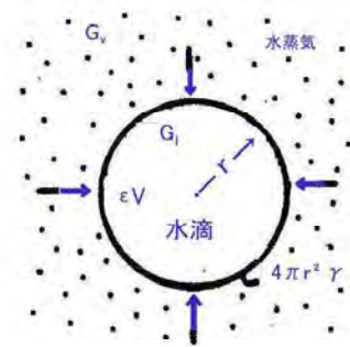
図 5.3 水滴の発生
