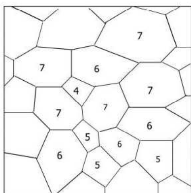
図 1.26 多結晶氷の断面
