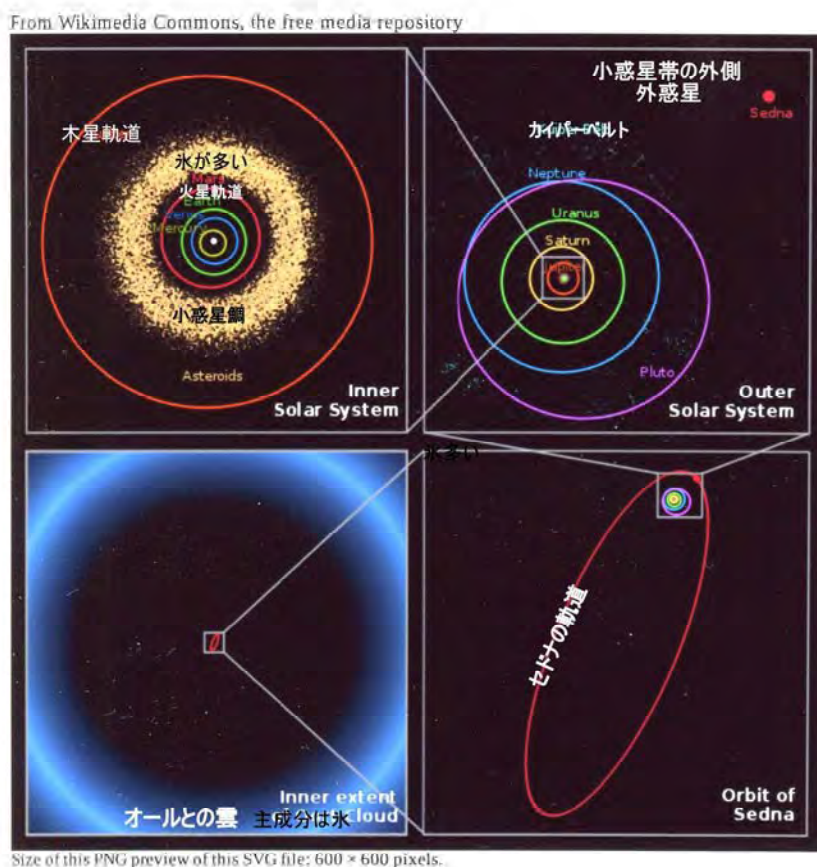
図 1.31 太陽系宇宙の氷
