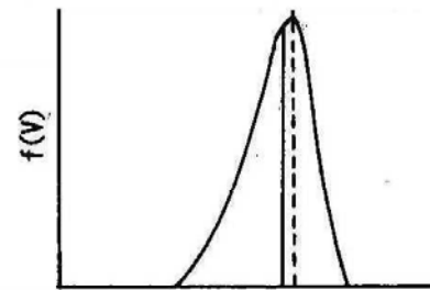
図 4.10 分子の運動
