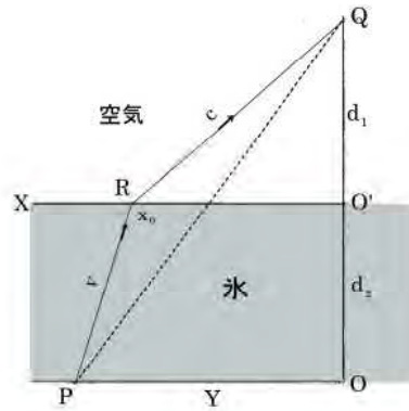
図 2.28 氷による光の屈折
