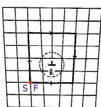
図 3.24 刃状転位
