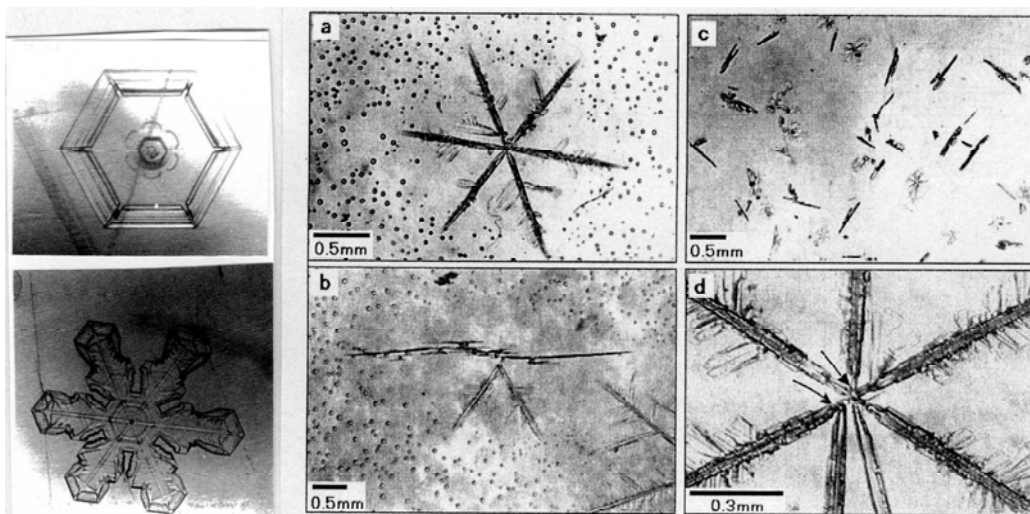
図 5.34 油川式人工雪作成法とケース内に成長した雪結晶
