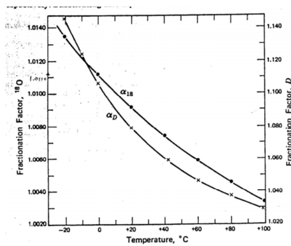
図 8.2 水と水蒸気間の分配係数
