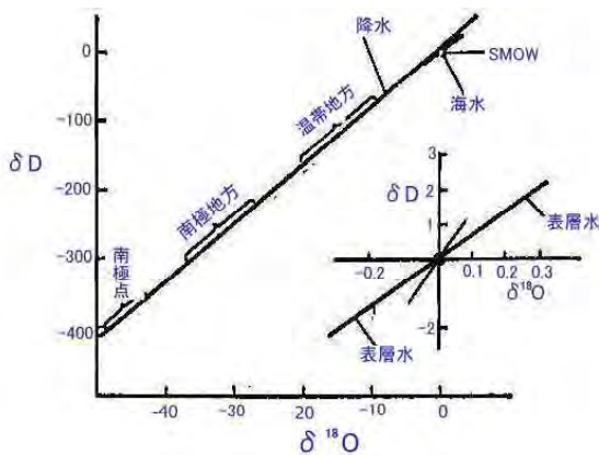
図 8.3 \delta^{18}\text{O} と \delta\text{D} の関係
