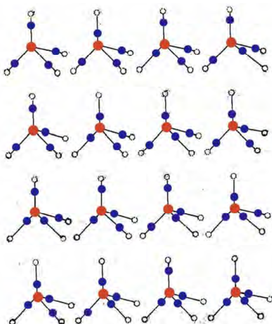
図 1.25 酸素原子の周りの水素原子の配置の数と水分子の構成数 (16 通り)
