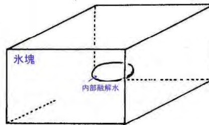
図2.22 負圧の発生
