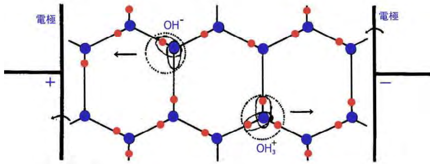
図 2.33 氷の中のイオン
