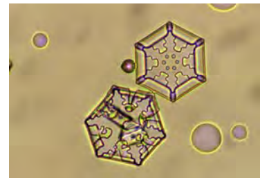
氷晶
