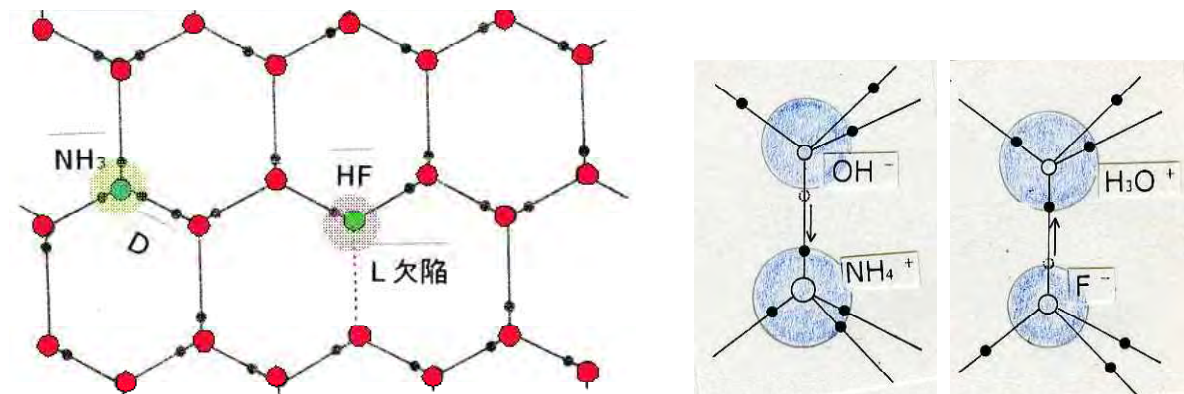
図 1.20 不純物による点欠陥
