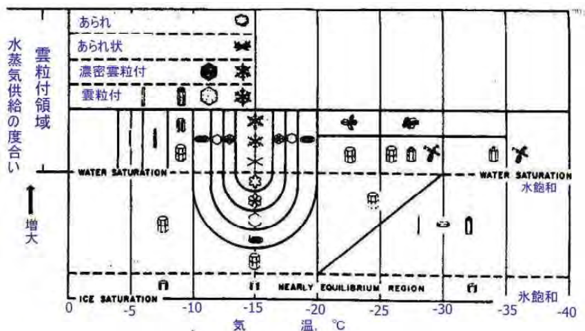
図 5.31 孫野による雪結晶の分類図表
