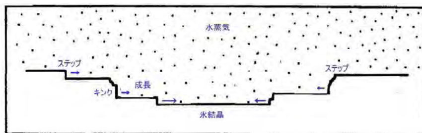
図 5.6 ステップの成長
