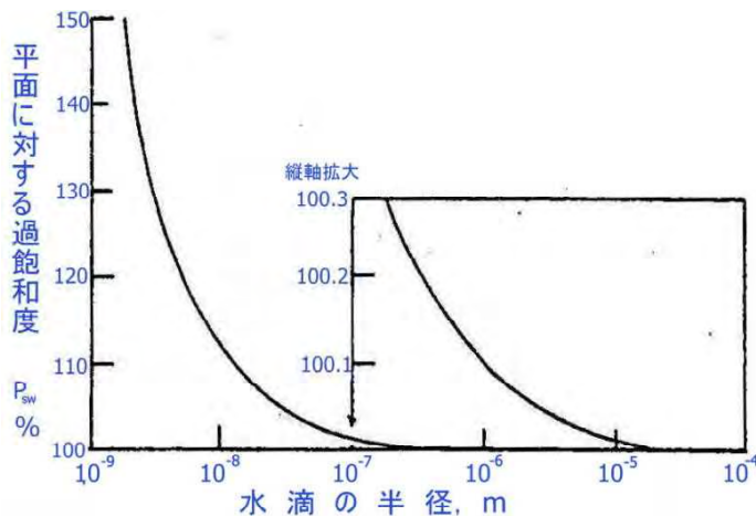
図 4.4 水滴の半径と過飽和度
