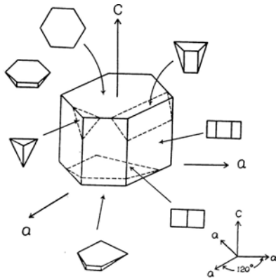
図4.8 蒸発ピットの形
