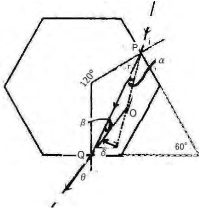
図 6.24 頂角 60 度面のフレの角
