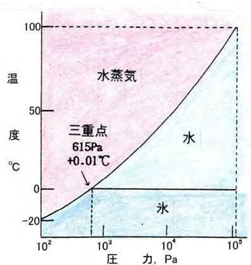
図 1.21 氷の状態図
