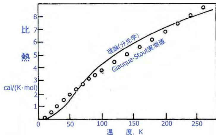
図 4.1 氷の比熱
