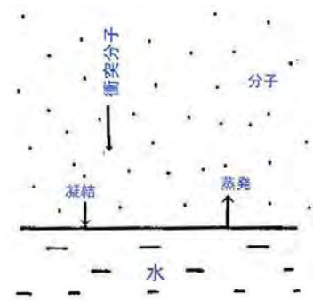
図 4.9 水の蒸数 \alpha は発と凝結
