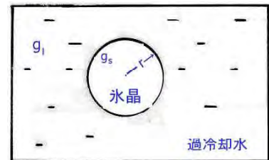
図 5.4 過冷却水中の氷晶
