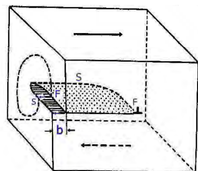
図 3.25 らせん転位
