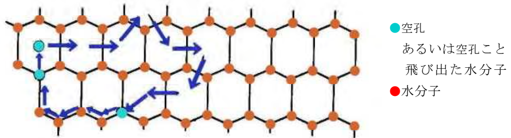
図 1.16 氷の内部での分子(格子間分子)の移動
