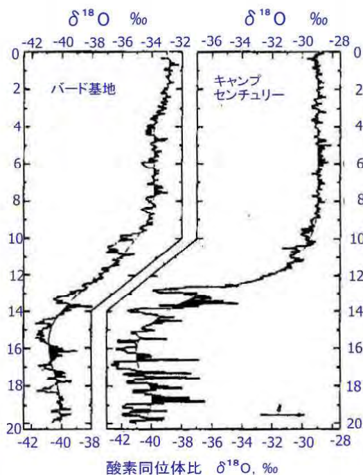
図 8.5 南極とグリーンランドの氷の \delta^{18}\text{O} と年代
