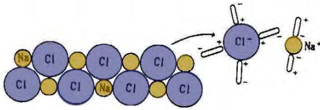
図 1.4 NaCl の水への溶解
