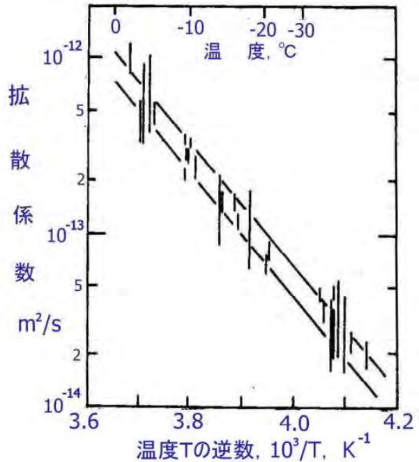
図 2.16 氷の自己拡散係数 (Onsager and Runnels, 1963)
