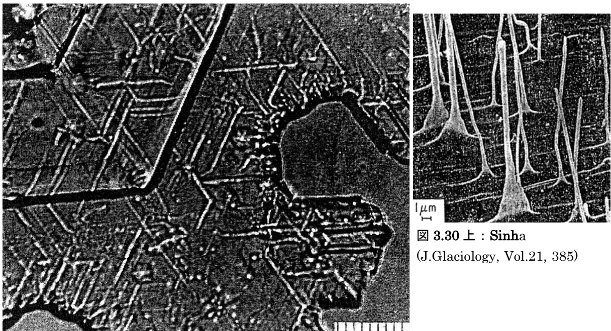
図3.29 結晶表面にできた転位チャネル (黒岩大助による)
