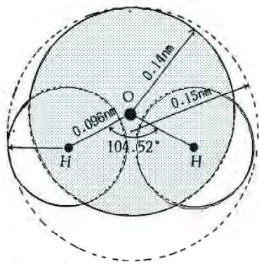
図1.1 水分子
