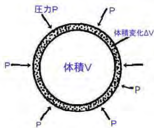
図 2.21 静水圧による収縮
