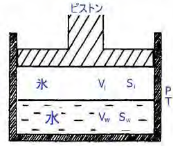
図 4.6 圧力融解
