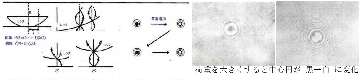
図 6.14 氷の表面に出来たニュートンリング（荷重を変えている）
