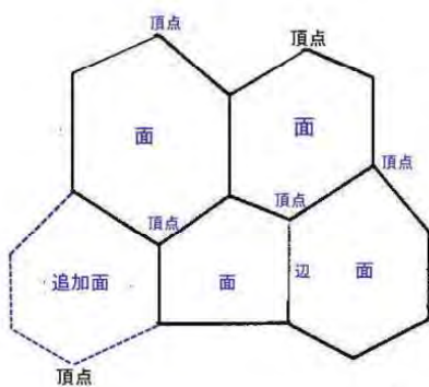
図 1.29 氷の切断面
