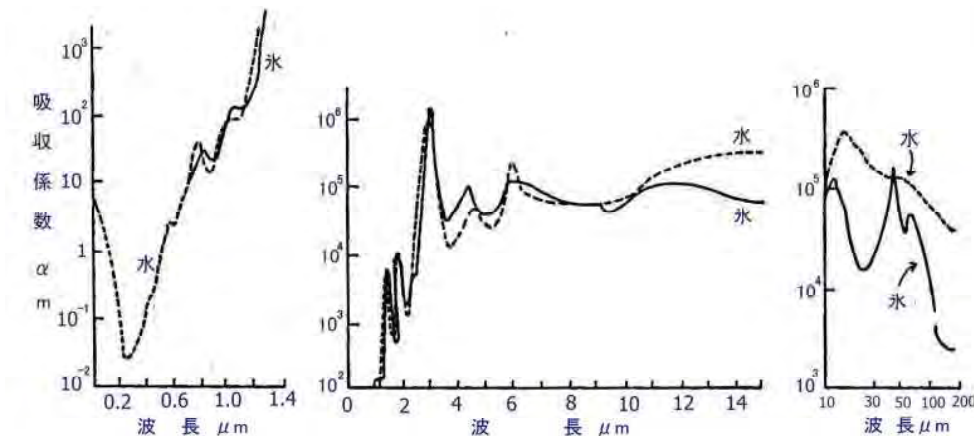
図 6.7 波長による光の吸収
