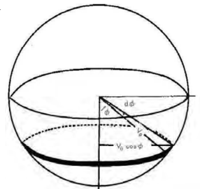
図 4.10 分子の運動
