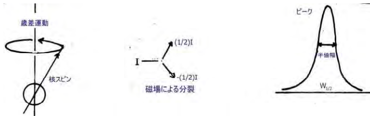
図 6.22 磁気共鳴
