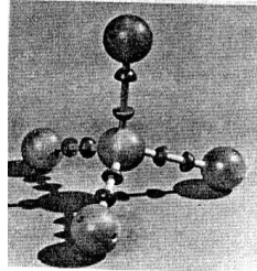
図 1.5 氷の四面体模型
