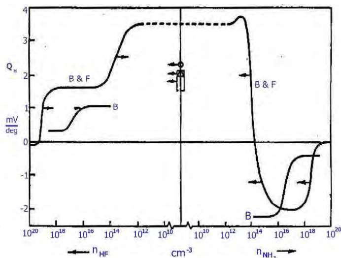
図 7.22 氷の熱電能 Q_H , mV/K
