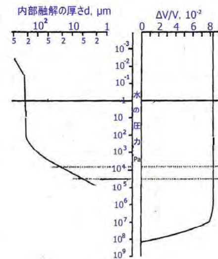
図 4.18 内部融解水の圧力
