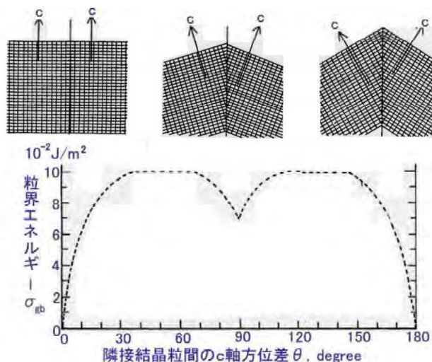
図 2.13 氷の結晶粒間の粒界エネルギー (鈴木重尚, 低温科学, 1970)
