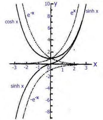
図 3.19 \sinh x と \cosh x および e^x と e^{-x}
