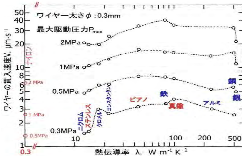
図 4.28 ワイヤーの貫入速度 v とワイヤーの熱伝導率 \lambda の関係
