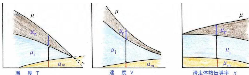
図 3.54 熱解析による温度 T , 速度 v , 滑走体熱伝導率 k の効果 (Evans et al. 1976)
