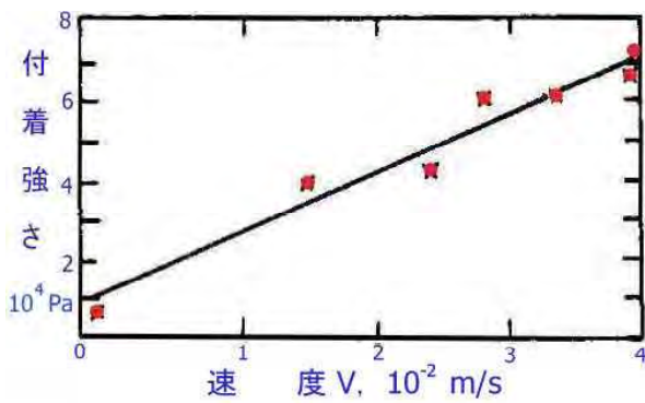
図 3.42 オプティカルフラットな水晶とゆき氷の付着強さ(Jellinek, 1960)
