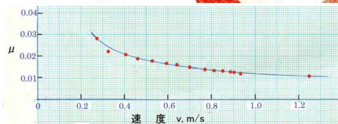
上：カール 下：カーリング・ストーンの速度と摩擦係数
