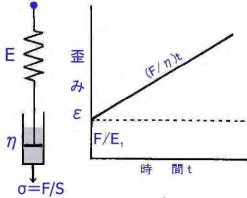
図 3.3 マックスウェル(Maxwell)要素
