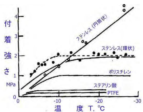
図 3.41 氷に対するステンレスおよびプラスチックの付着強さ(Raraty & Tabor,1958)
