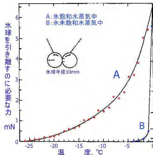
図 3.B 氷球間の付着実験と付着力の測定結果 (中谷・松本)
