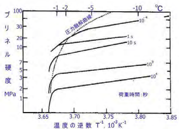
図 3.23 氷のブリネル硬さ(Barnes et al.1971)
