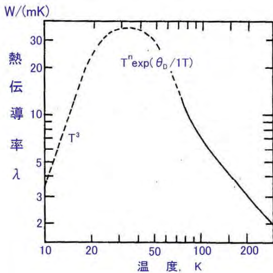
図 2.9 氷の熱伝導率の温度依存性 (フレッチャー著(前野紀一訳)氷の物理化学(共立出版))
