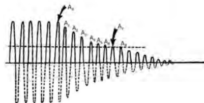
図3.33 強制振動から自由振動（減衰振動）に移行したときの振動（振幅）減衰の変化
