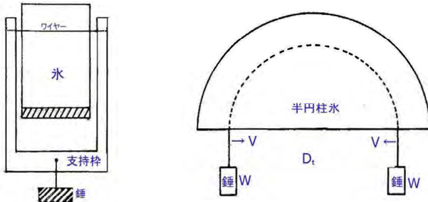
図 4.25 融けつつある氷へのワイヤーの貫入(左：定常法, 右：非定常法)
