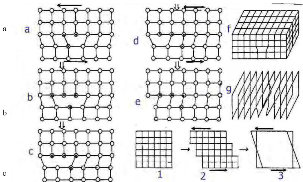
図 3.26 剪断力を受けたとき、刃状転位による結晶の変形過程
