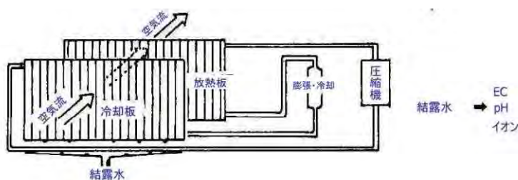
図 8.12 除湿器による大気環境計測
