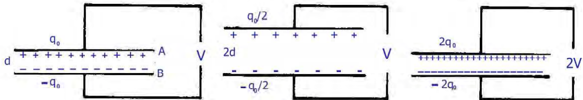
図 7.11 コンデンサー (a) 間隔 d , 起電力 V ; (b) 間隔 2d , 起電力 V ; (c) 間隔 d , 起電力 2V コンデンサーの容量 C = (1/4 \pi \epsilon_0) (S/d) , q = CV = (S/4 \pi \epsilon_0) (V/d) S は電極の面積, d は電極の間隔
