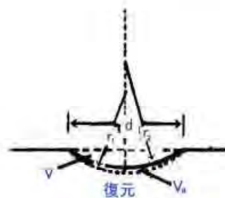
図 3.59 球と平板の衝突
