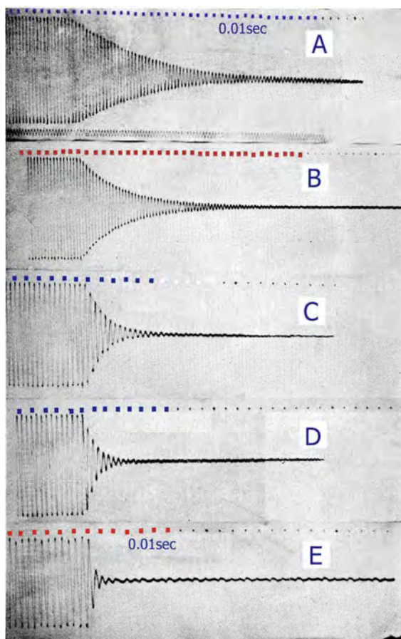
図3.33 強制振動から自由振動（減衰振動）に移行したときの振動（振幅）減衰の変化
