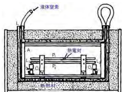
図 3.31 内部摩擦測定装置
