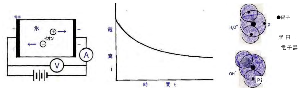
図 7.2 氷を流れる電流の測定
