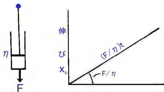
図 3.2 ダッシュポット（完全塑性体）
