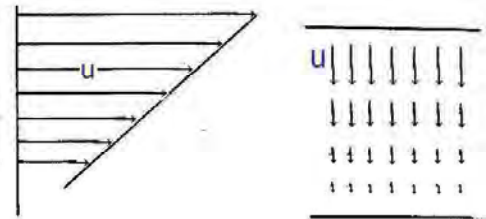
図 3.16 液体の流れ（左）と積雪の圧縮（右）
