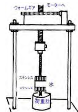
図 3.38 ジェリネックの付着力測定装置(Jellinek, 1953)
