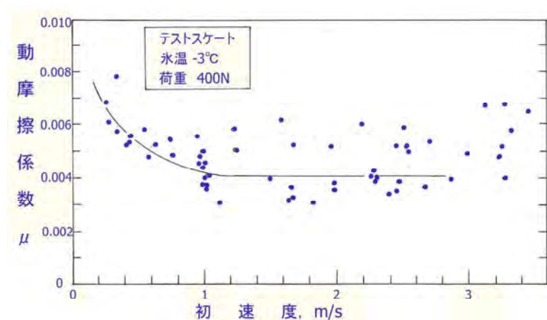
図 3.51 スケート(スピードスケート)の初速と平均摩擦係数
