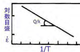
図 3.18 活性化エネルギー 歪み速度 \dot{\epsilon} と 1/T
