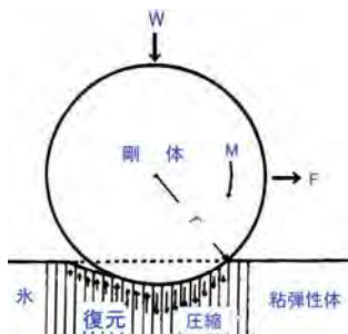
図 3.54 ころがり摩擦
