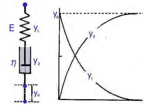
図 3.6 一定歪みを与えられたマクスウェル要素
