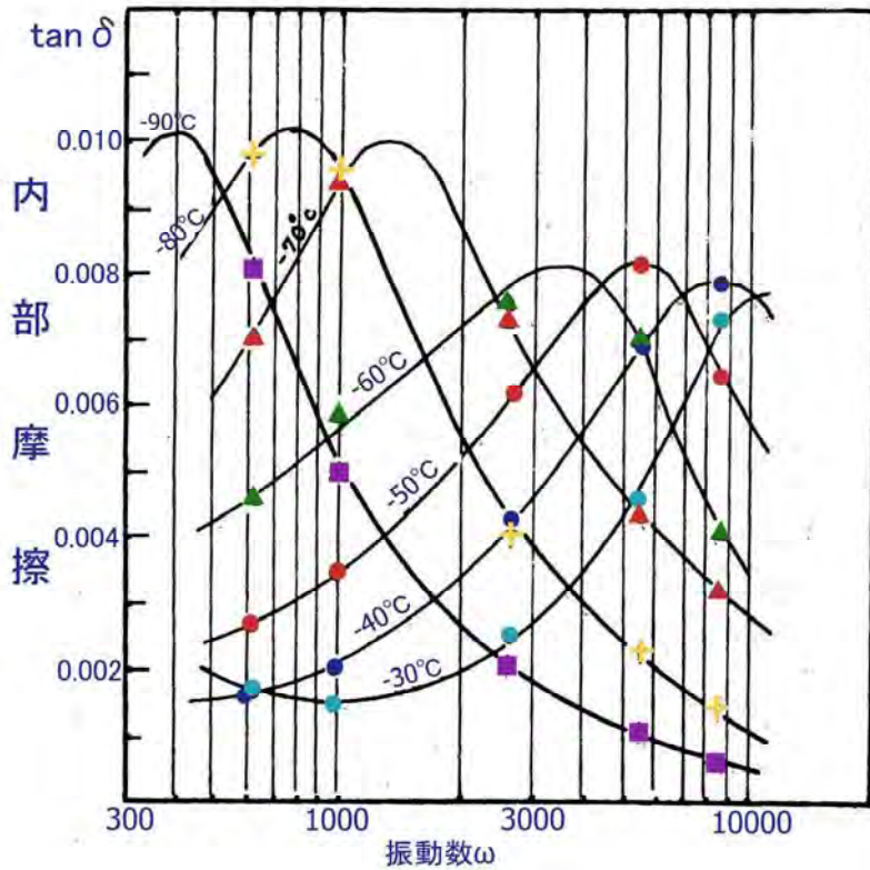
図 3.34 氷の内部摩擦の周波数 \omega 依存性 (黒岩・山地, 1959)
