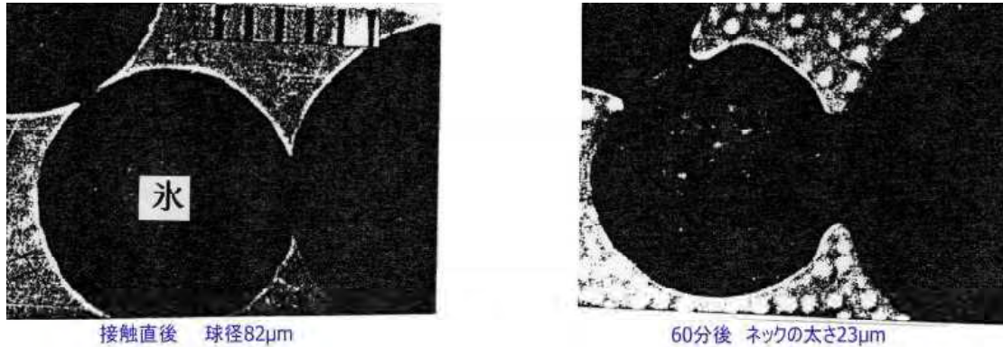
図 4.13 氷同士の焼結(黒岩, 1960)
