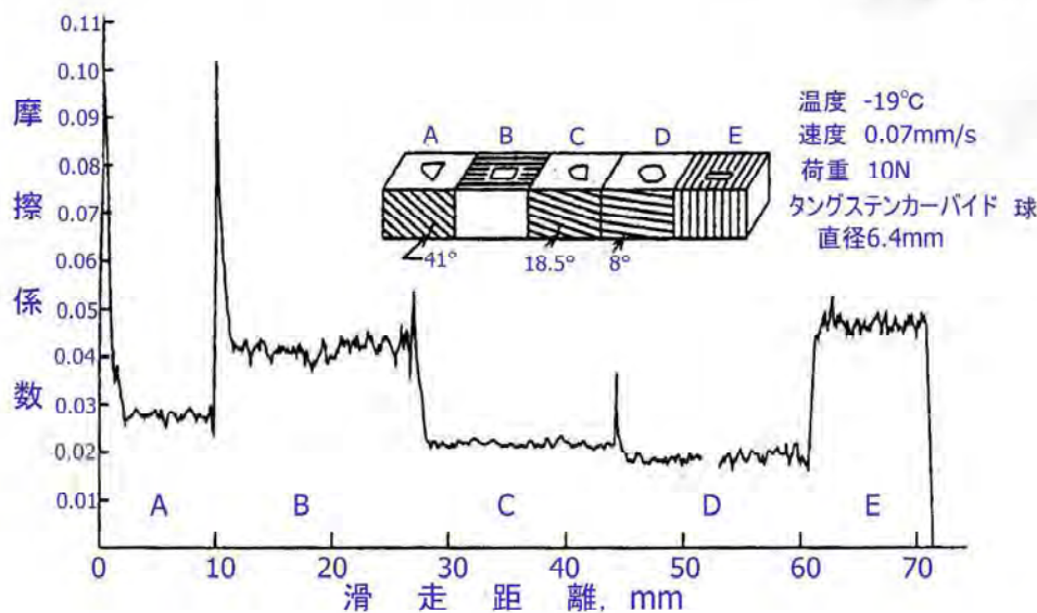
図 3.47 結晶面による摩擦の違い
