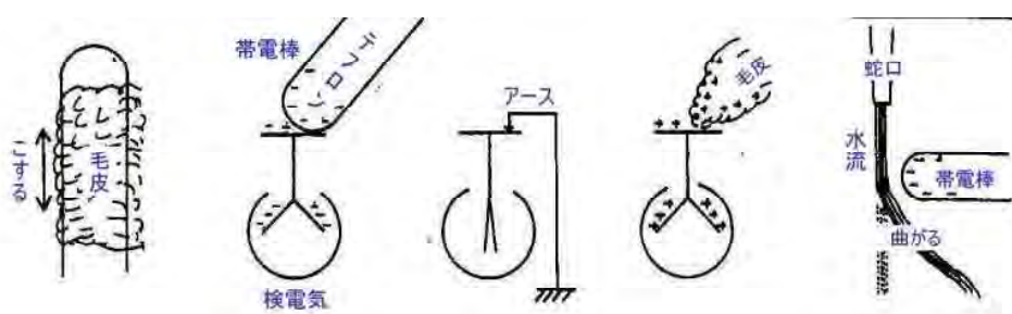
図 7.14 帯電と検電器
