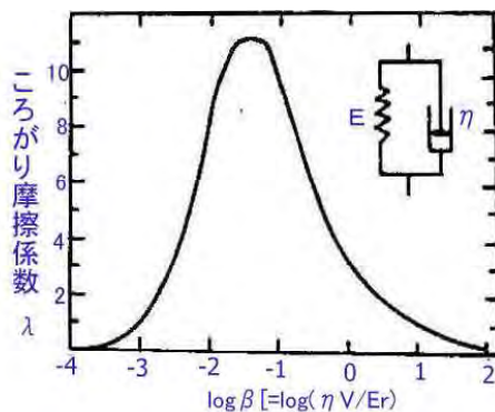
図 3.55 ころがり摩擦係数の速度依存性(Flom et al.,1959)
