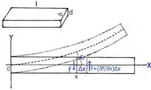
図 A.1 一端を固定された棒の撓み
