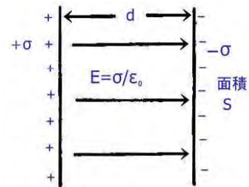
図 7.12 \sigma , E , S , d
