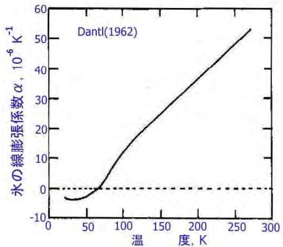
図 2.3 氷の線膨張係数
