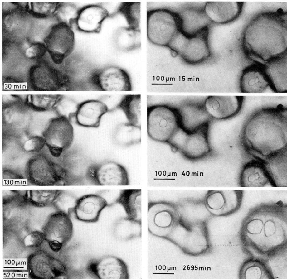
図 4.16 左：ガラス板と氷球の付着，右：氷板と氷球の付着（水野，低温科学 1979）
