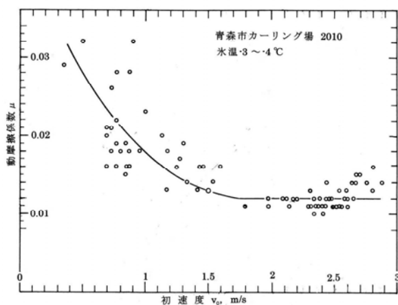
カーリング・ストーンの摩擦係数
