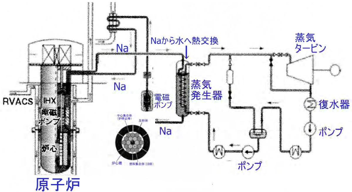
4S 小型原子炉の構成図（太田・福永：小型高速炉 4S と高速炉技術．東芝レビュー，65，No.12）
