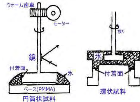
図 3.40 Raraty & Tabor の実験法(1958)
