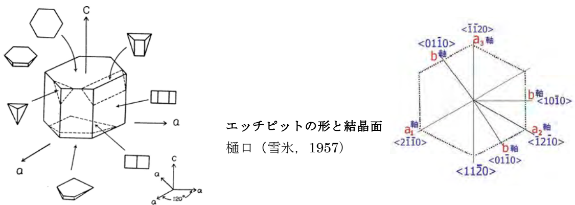
図 1.9 結晶面の指数表示 (平行な面は同一指数で表示される)
