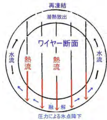
図 4.26 熱流
