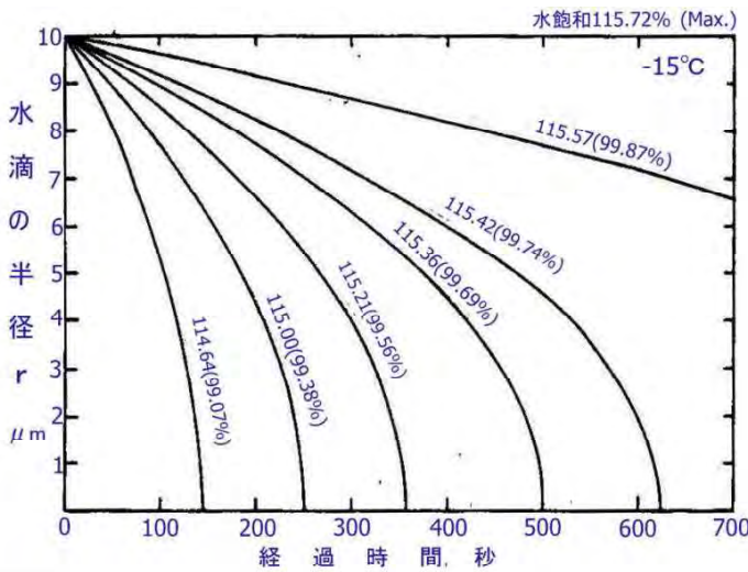
図 5.35 油川式人工雪作成装置における 拡散場の水滴の消失過程 (環境相の水蒸気密度をパラメーターとした)
