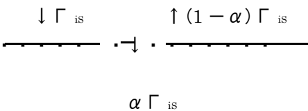
図 4.2 水の蒸発と凝縮
