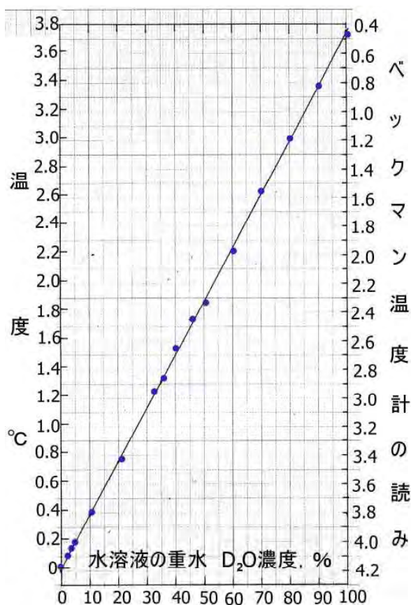
図 2.34 重水水溶液の氷点
