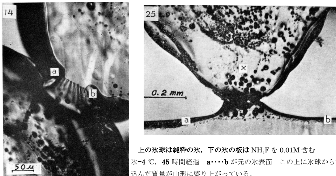
図 4.15 純氷球間の焼結,
