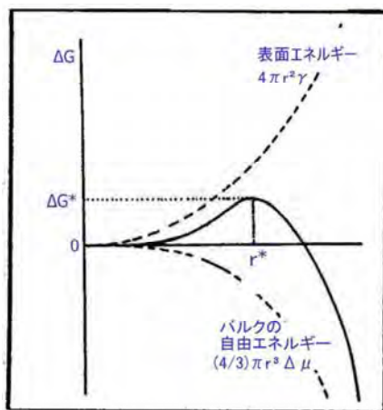
図 5.2 結晶の臨界半径
