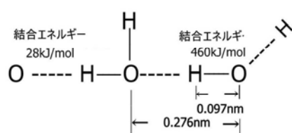
図 1.11 水分子の水素結合
