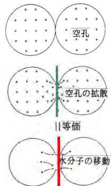
図 1.15 氷の焼結
