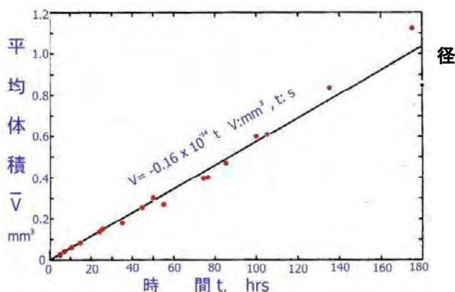
図 5.26c 経過時間 t と雪粒の平均体積
