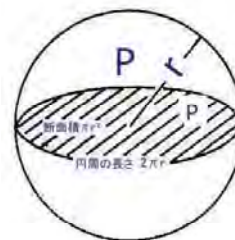
図 2.12 表面張力の説明図
