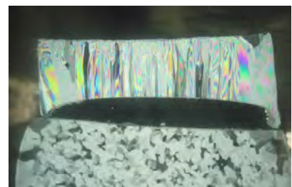
水槽の水の凍結 上：鉛直断面、下：水平断面
