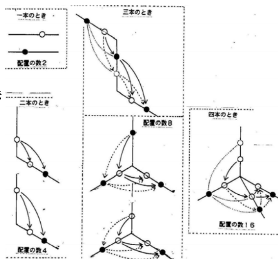
図 1.24 結合線上に水素原子
