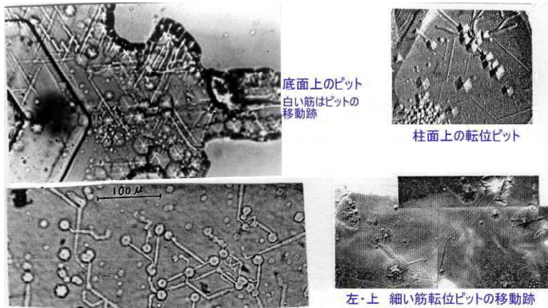
図 4.12 氷の転位ピット(黒岩大助)
