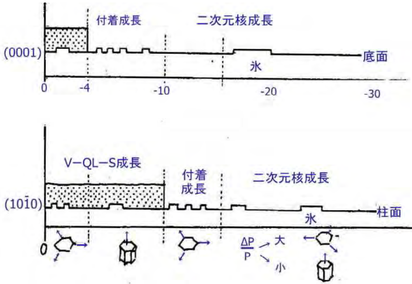
図 5.11 氷の底面 (0001) と柱面 (10 \bar{1}0 ) の表面状態 (黒田)
