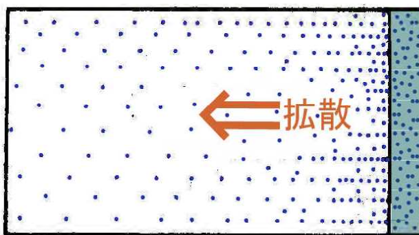
図 1.14 氷内部の異物の拡散
