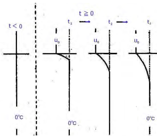
図 5.22 湖水の凍結
