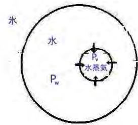
図 4.17 内部融解
