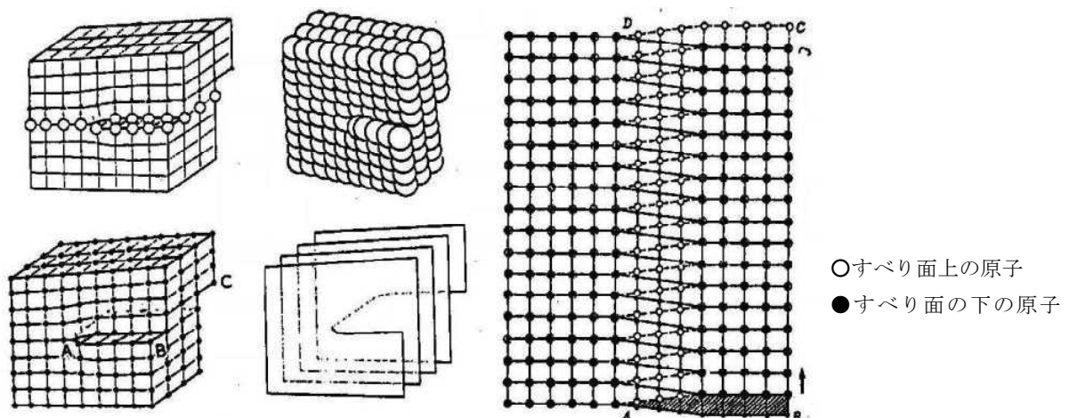
図 3.27 らせん転位
