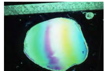
氷箭の水平断面 差し渡し 100mm の巨大な 単結晶だった
