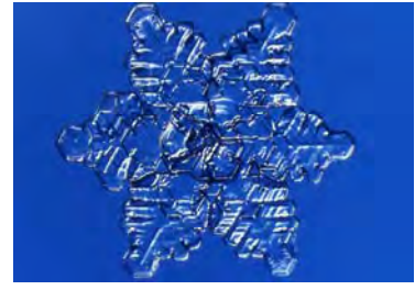
広幅六花結晶
