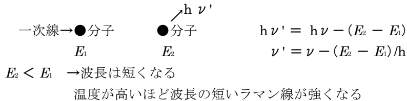
図 6.21 ラマン分光
