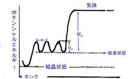
図 5.7 分子のポテンシャル
