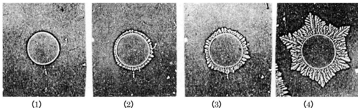
図 5.23 円盤氷の成長(荒川淳)
