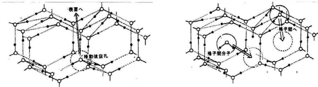
図 1.33 左：Schottky 欠陥(空孔形成) と右：Frenkel 欠陥(空孔と格子間分子の対形成)
