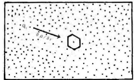
図 5.13 過飽和水蒸気中での氷の成長
