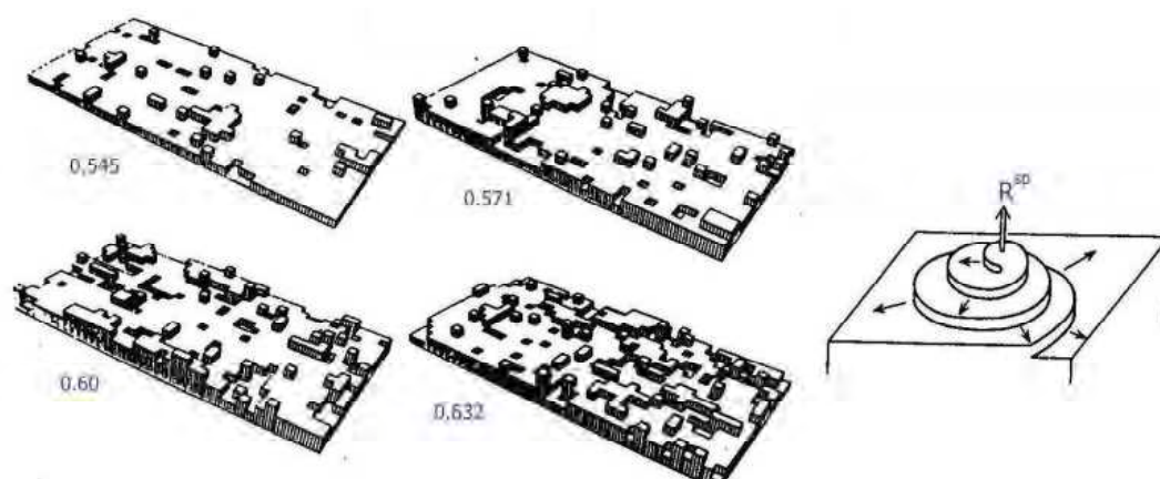
図 5.5 分子オーダーから見た氷表面の構造（黒田「結晶は生きている」より転載）
