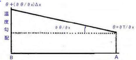
図 2.8 温度勾配の変化
