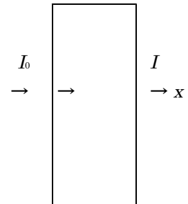
図 6.6 光の吸収
