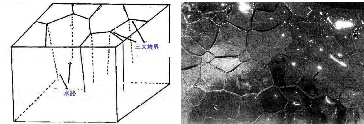
図 4.21 氷の中の水路（写真の多角形は結晶粒の表面，水路ではない）
