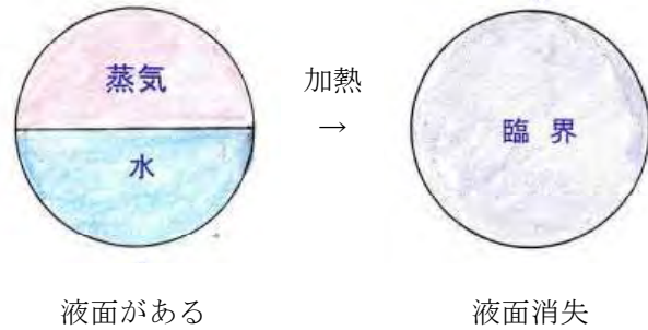
図 1.22 臨界 ( 374^\circ \text{C} , 22 \text{ MPa} )
