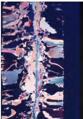
つららの鉛直断面 多結晶
