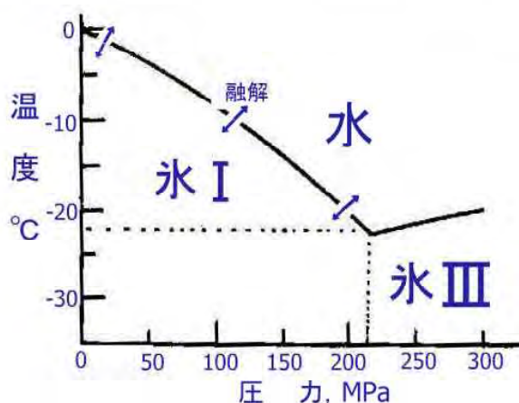
図 2.2 氷の状態図
