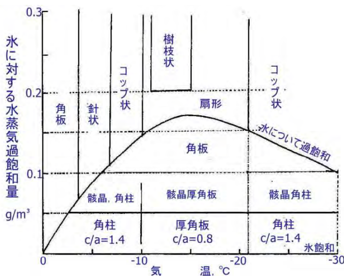
図 5.33 小林のダイヤグラム (雲のない空間で作られた結晶分類)
