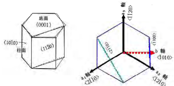
図 1.8 結晶方位< >と面記号 ( )
