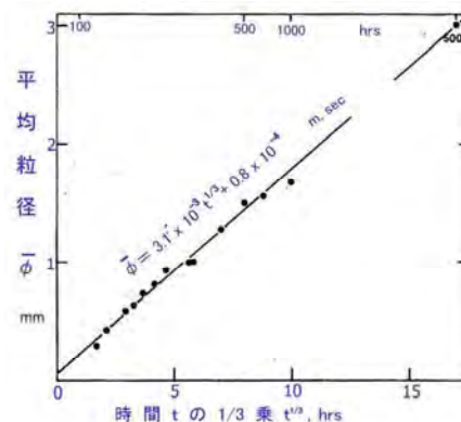
図 5.26b 経過時間と雪粒の平均粒径
