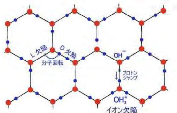
図 1.18 D, L 欠陥とイオン欠陥( OH_3^+ , OH^- )
