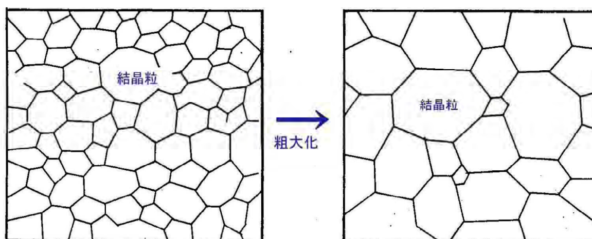
図 5.27 結晶粒の粗大化 左：N=75，右：N=28（3 倍に粗大化）
