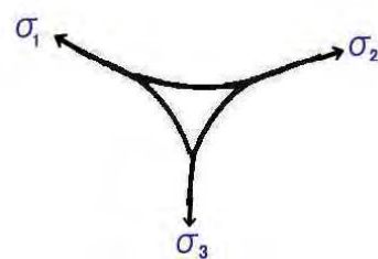
図 2.14 三叉境界の釣り合い
