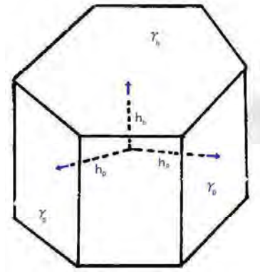
図 5.24 氷の平衡形
