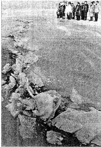
図 2.5 お神渡り
