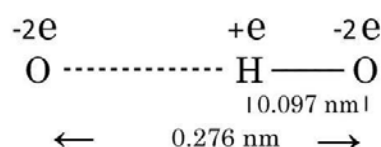
図 1.12 水素結合における電荷分布模型
