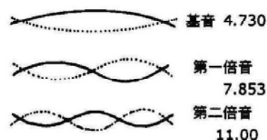
振動模式と m
