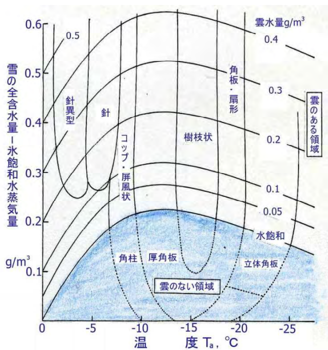
図 5.30 中谷ダイヤグラム
