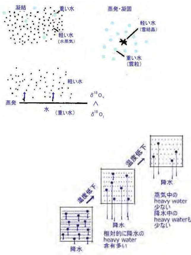
図 8.1 \delta^{18}\text{O} , \delta\text{D} の変化
