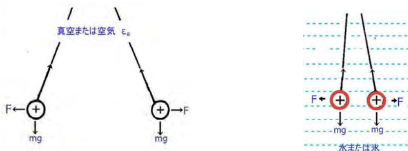
図 2.32 誘電率
