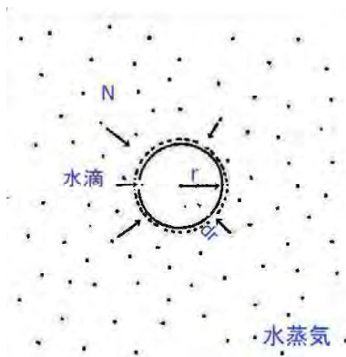
図 4.3 液滴の蒸気圧
