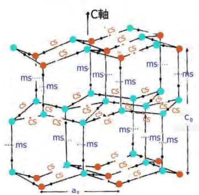
図 1.5 氷の四面体模型
