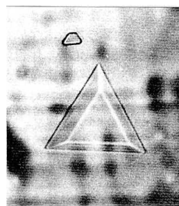
図 1.30 クラスレート氷 (雪氷辞典, 古今書院より転載)
