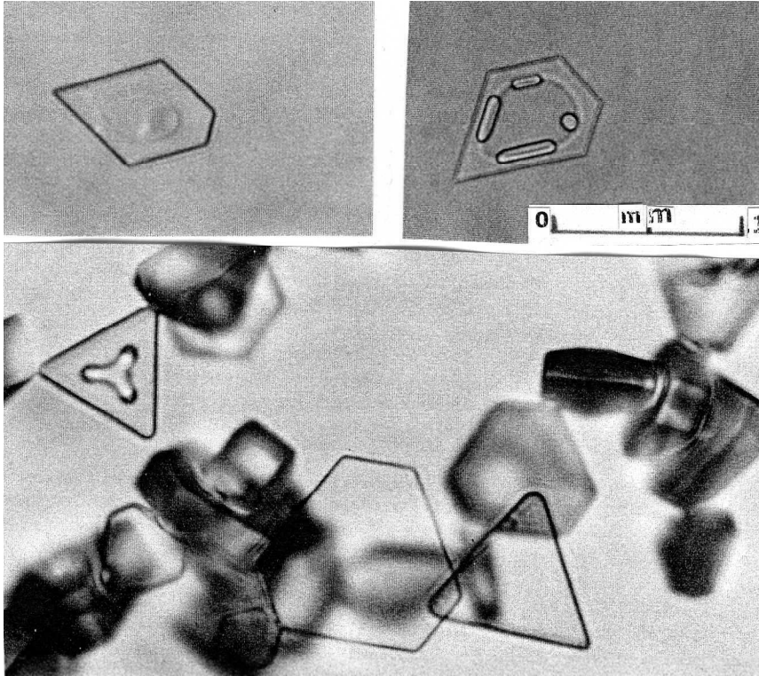
図 8.9 人工の酸性の雲(硝酸や硫酸を含む雲)から発生した奇形雪結晶
