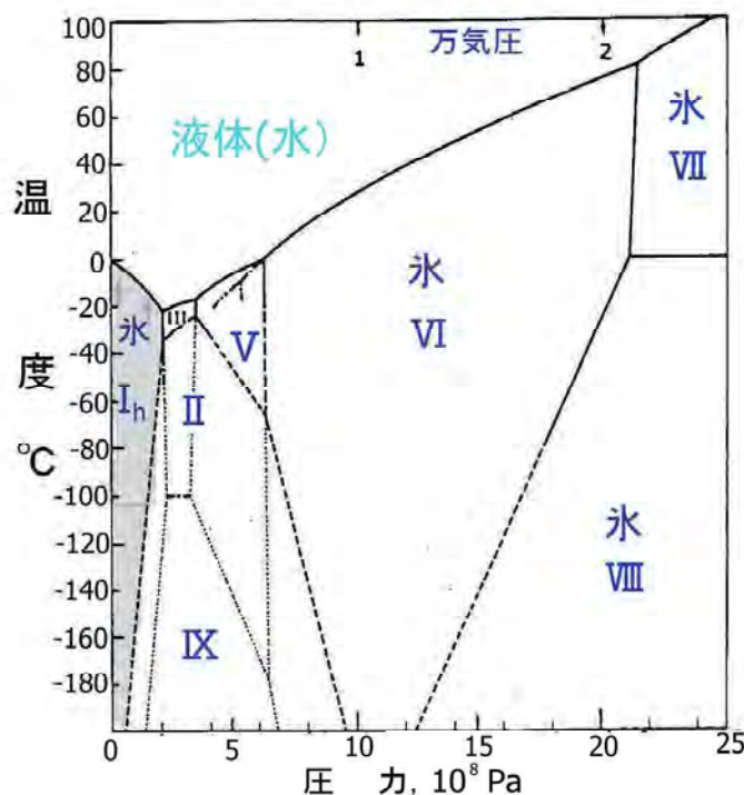
図 1.23 氷の多形
