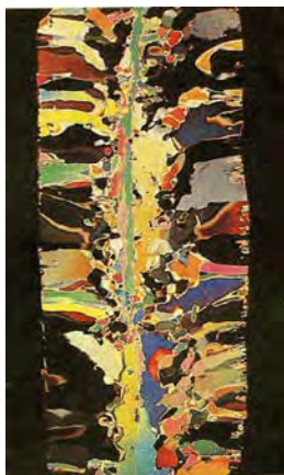
図 5.17 つらら (左) と氷筈 (右) の薄片 (鉛直断面)
