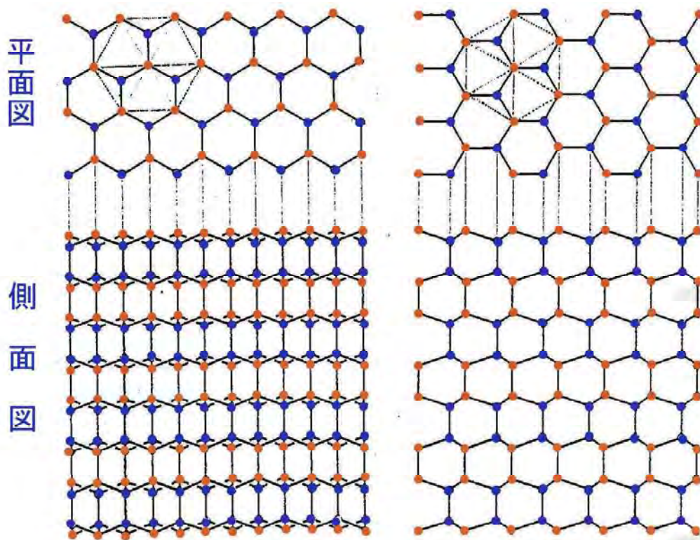
図 1.10 氷の結晶構造
