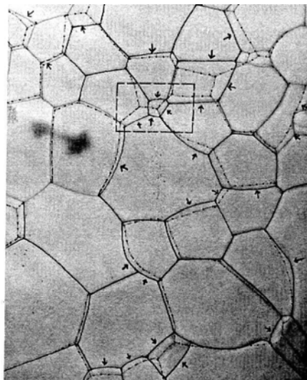
図 5.27 氷微結晶の成長
