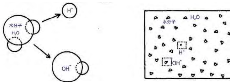
図 8.11 水分子から水素イオンと水酸イオンの形成
