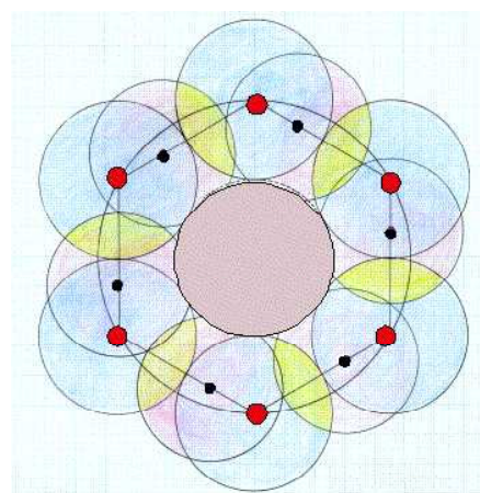
図 1.13 水素結合における電子雲の重なり (黄色)
