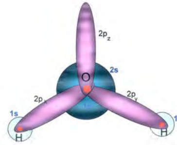
図 1.3 水分子の双極子
