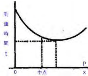
図 2.29 屈折点と到達時間の関係
