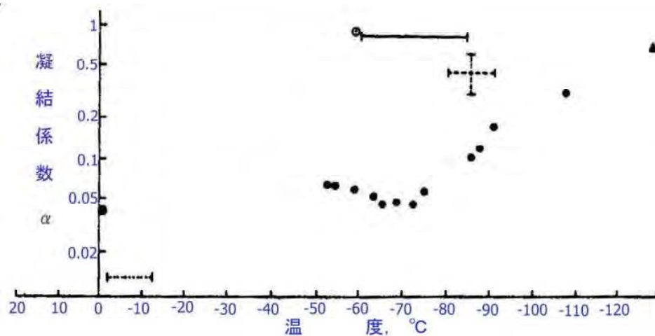
図 4.30 氷や水面に対する凝結係数 (P.V.Hobbs, Ice Physics. 1974, 443p より転載)
