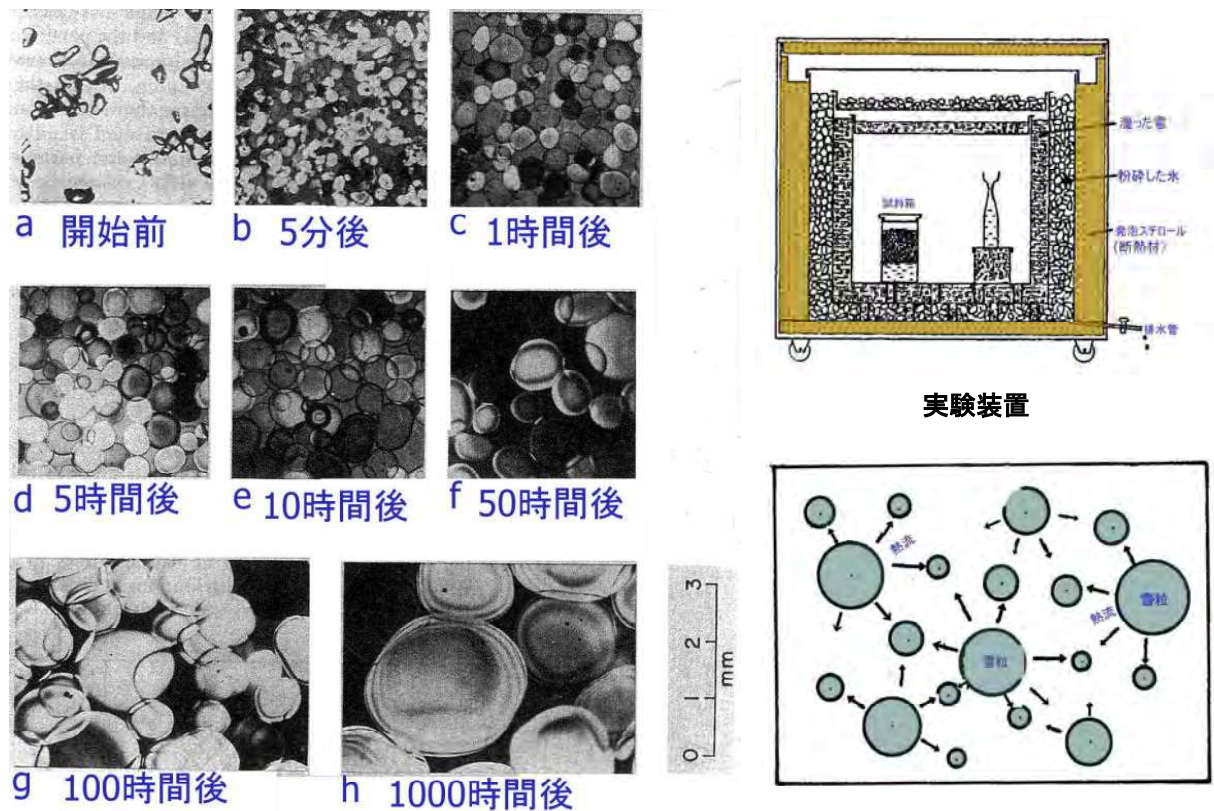
図 5.25 水に浸った雪粒の粗大化
