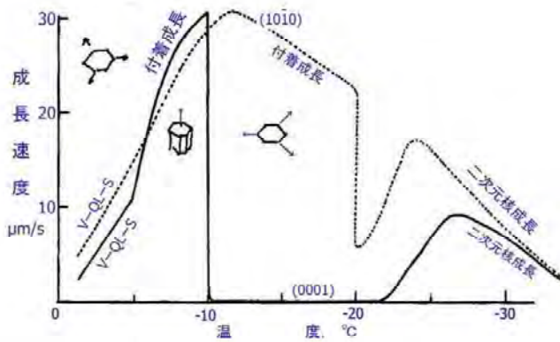
図 5.12 水飽和における (0001) 面の成長速度と (10 \bar{1}0 ) 面の成長速度の温度依存性 (黒田)
