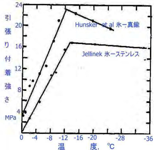
図 3.43 せん断付着強さの温度依存性(Jellinek)
