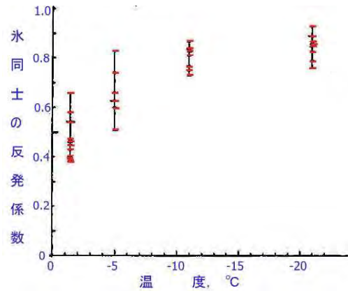
図 3.57 氷の反発係数の温度依存性 (同上より引用)
