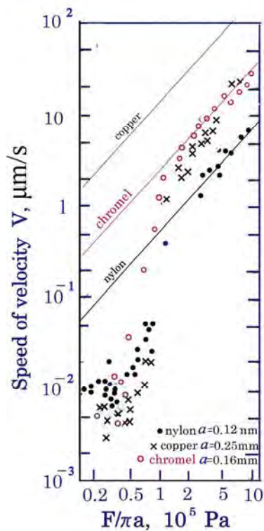
図 4.27 最大圧力 p_{\max} と貫入速度 v の関係 (Drake & Shreve, 1973)
