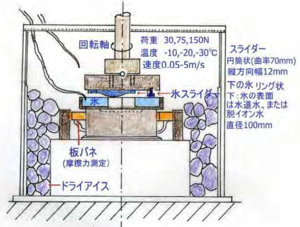
図 3.55 Akkok et. al. の実験装置
