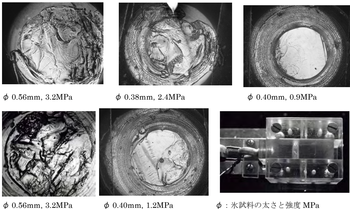
図 3.45 氷の剪断破壊面
