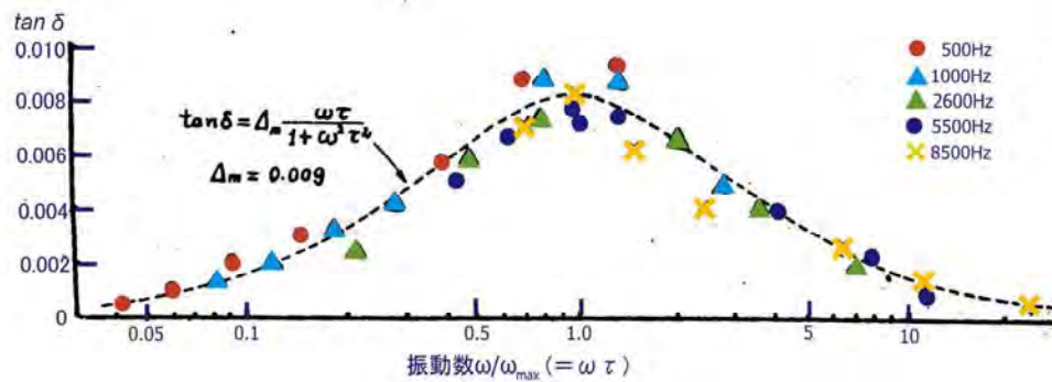
図 3.35 \tan \delta と \omega\tau の関係 (\tan \delta)_{\max} = 0.009
