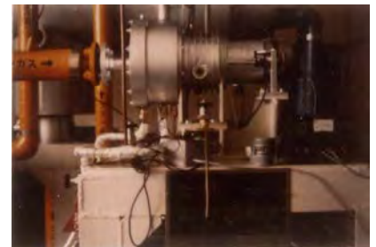
秋田大学で開発された雪を冷熱源とする温度差発電装置 右はフロン・タービンと発電機
